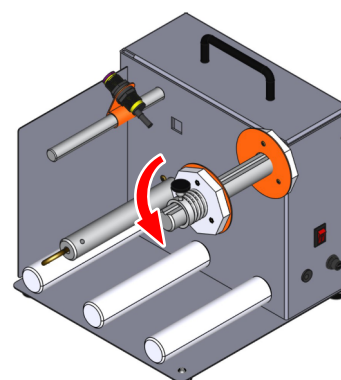
Sem tubete (Flanges-guia invertidas)
